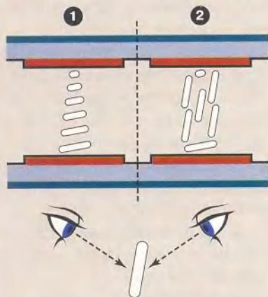
Рис. 1. ЖК-дисплеи с непостоянной цветопередачей
