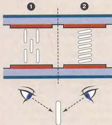
Рис. 2. ЖК-дисплеи с технологией VA
